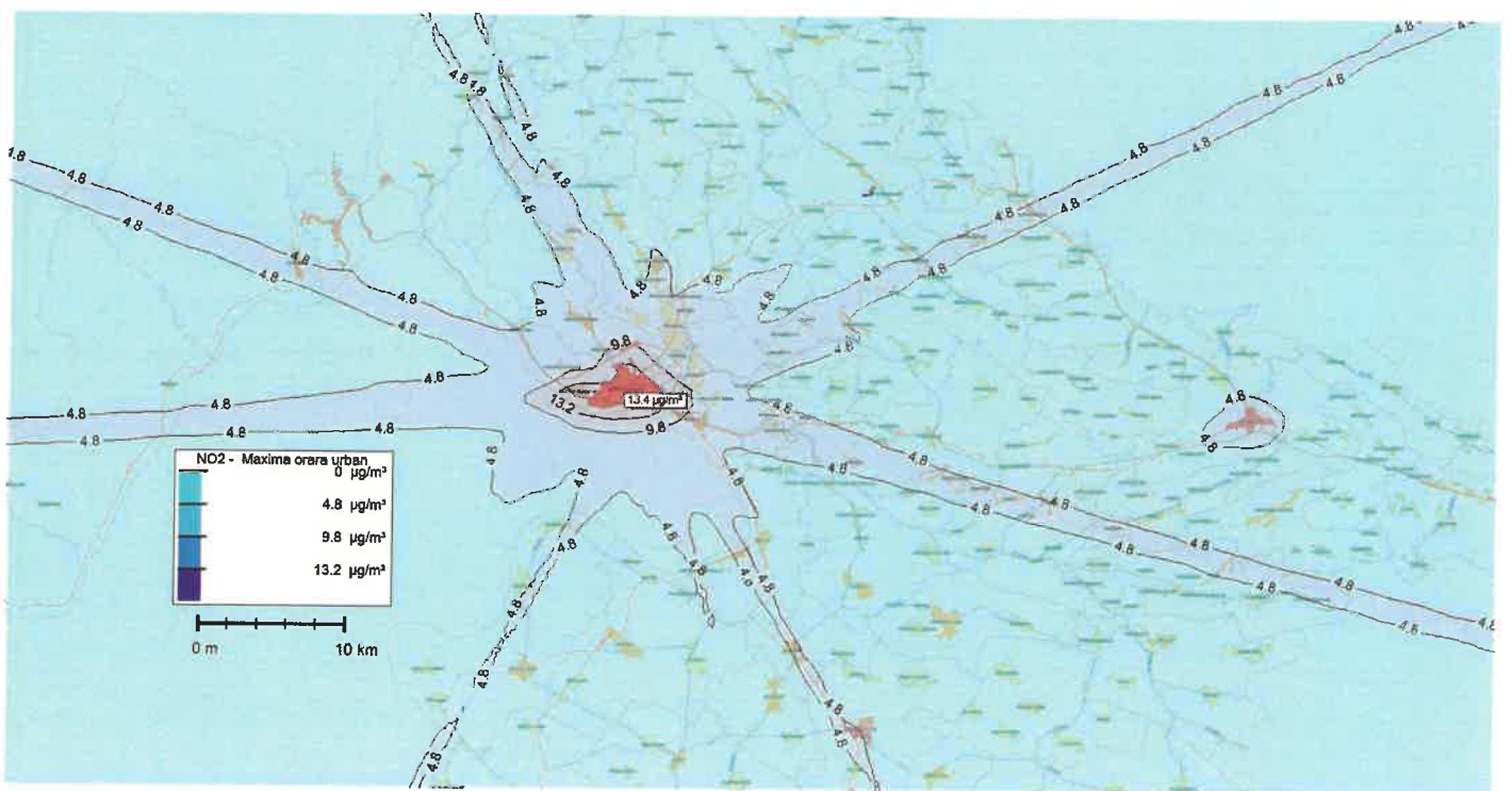
Anexa D.2.1.2.0 – Dispersia NO 2 în mediul urban din zona Mehedinti în anul de proiecție
