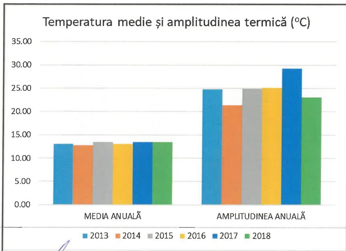
Figura B.4.2 – Evoluția temperaturilor medii anuale și a amplitudinii termice la stația Drobeta-Turnu-Severin în perioada 2013-2018
